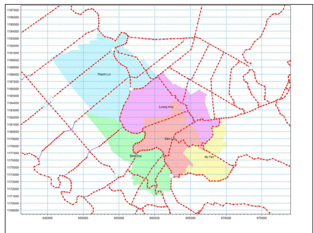
Hình 2. Mạng lưới tính toán thủy lực
