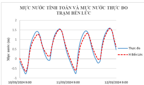
Hình 4. Kết quả hiệu chỉnh - kiểm định mực nước và lưu lượng tại trạm Bến Lức
