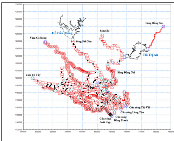
Hình 2. Mạng lưới tính toán thủy lực
