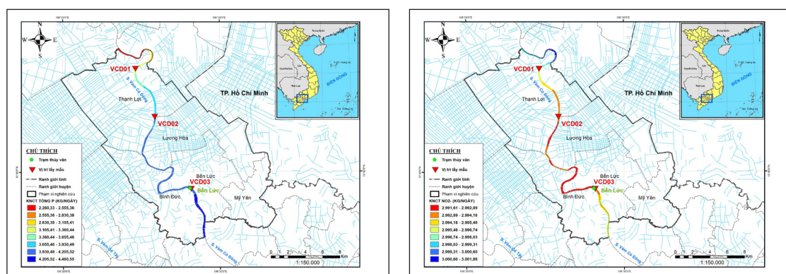
Hình 7. Khả năng chịu tải của nguồn nước Sông Vàm Cỏ Đông đoạn chảy qua khu vực Bến Lức: (a) Tổng P; (b) NO 2 -
