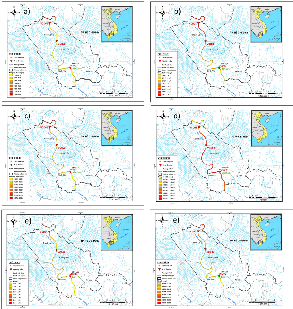
Hình 6. Biến đổi nồng độ các chất trong mùa khô: (a) \text{BOD}_5 ; (b) COD; (c) \text{NH}_4^+ ; (d) \text{NO}_2^- ; (e) Tổng N và (f) Tổng P
